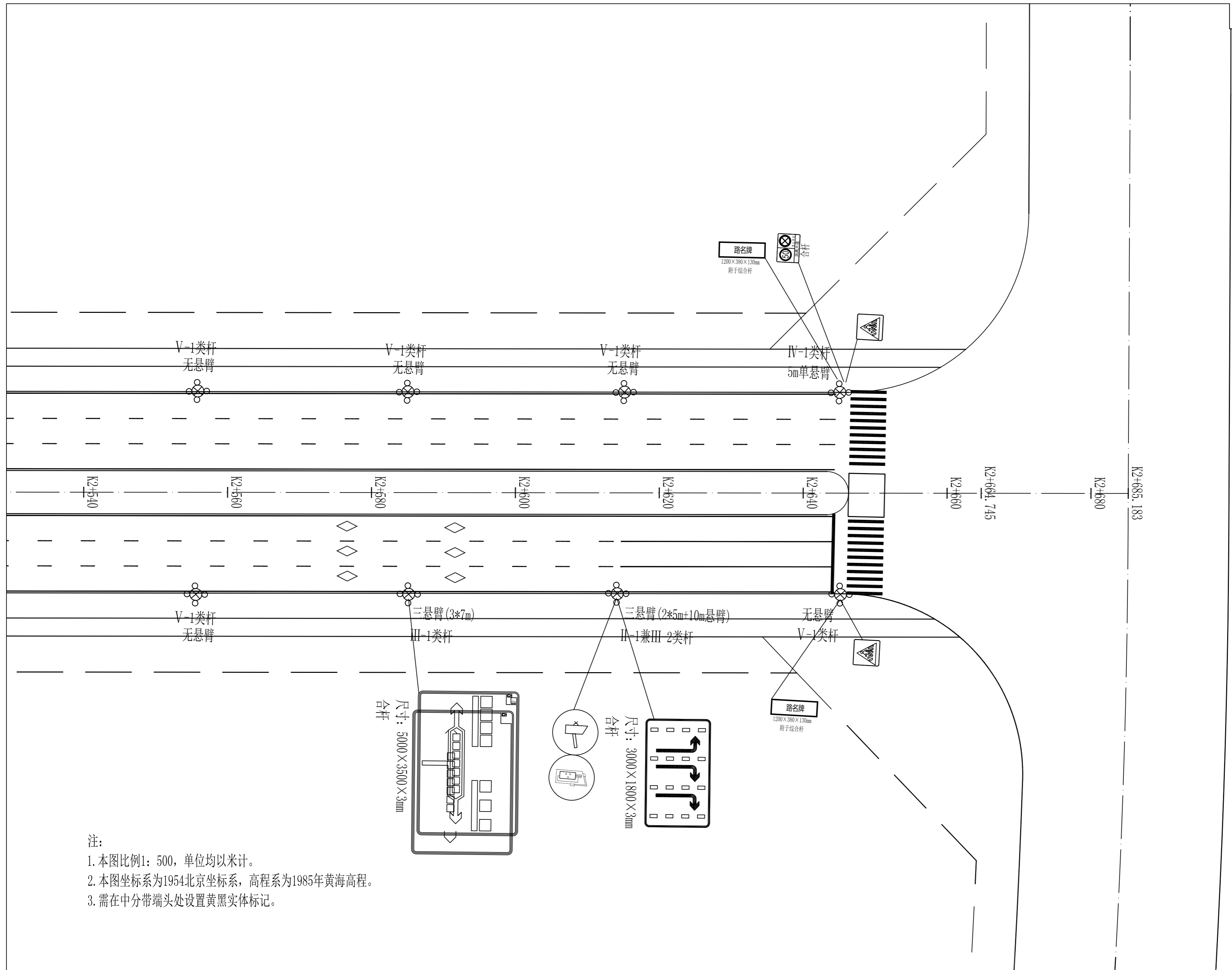
多杆合一平面设计图
