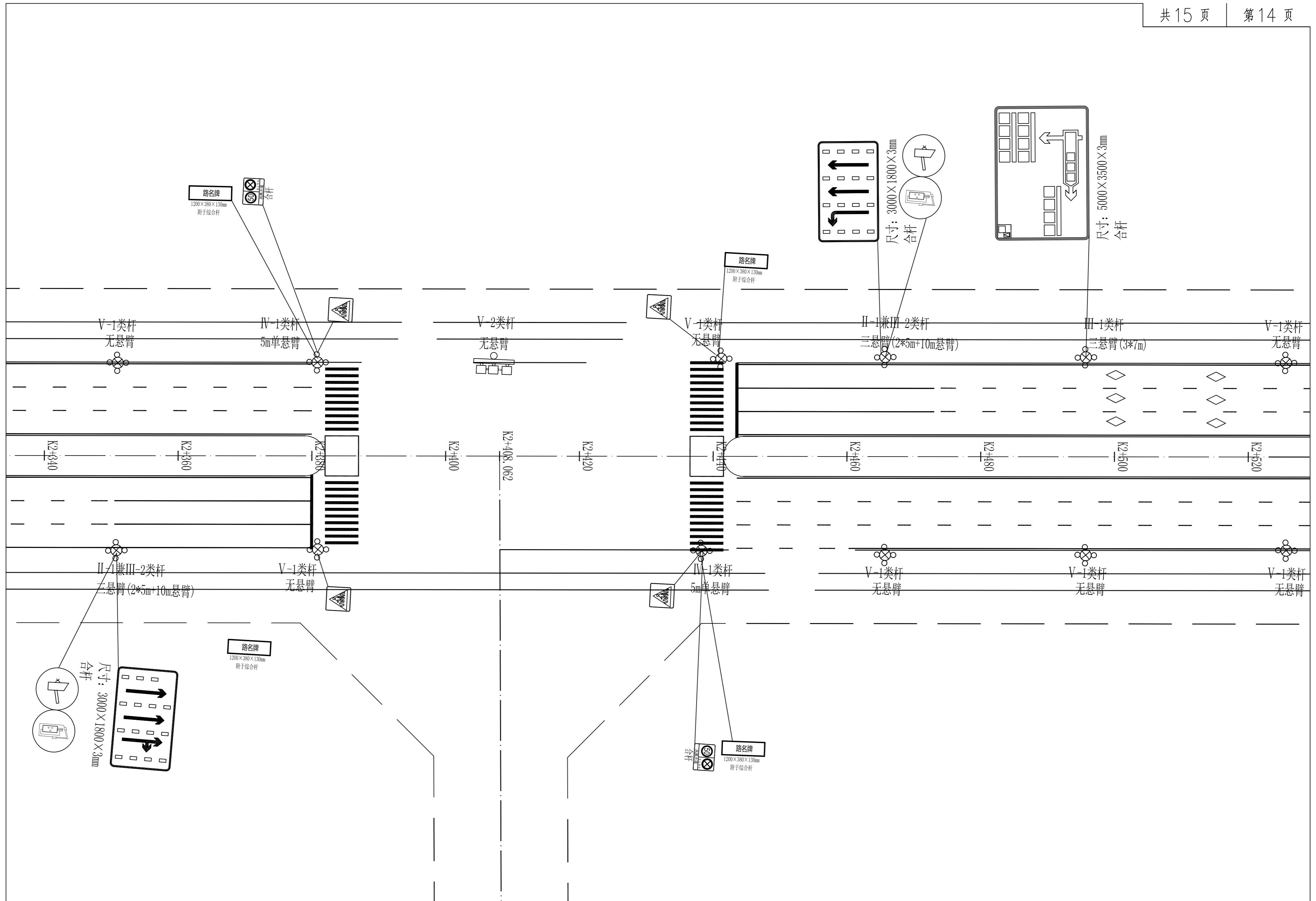
多杆合一平面设计图
