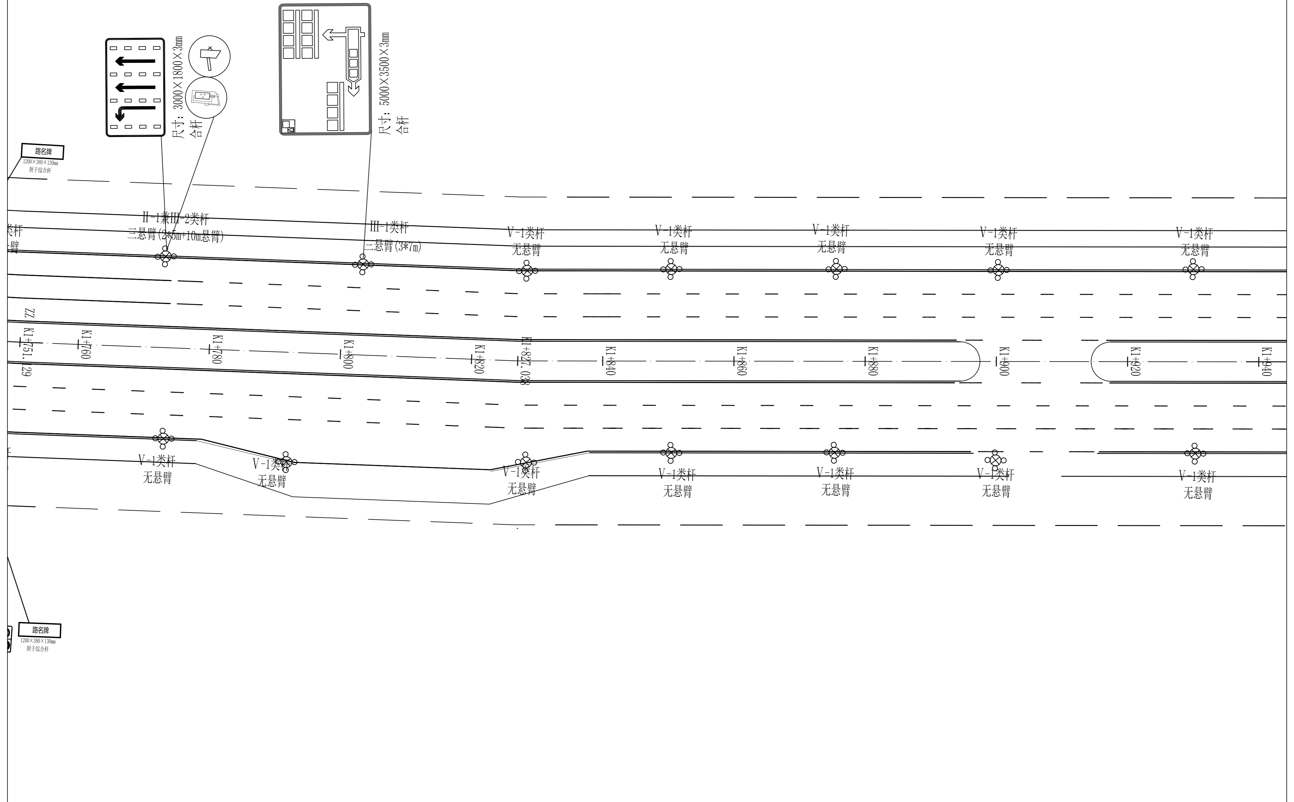
多杆合一平面设计图
