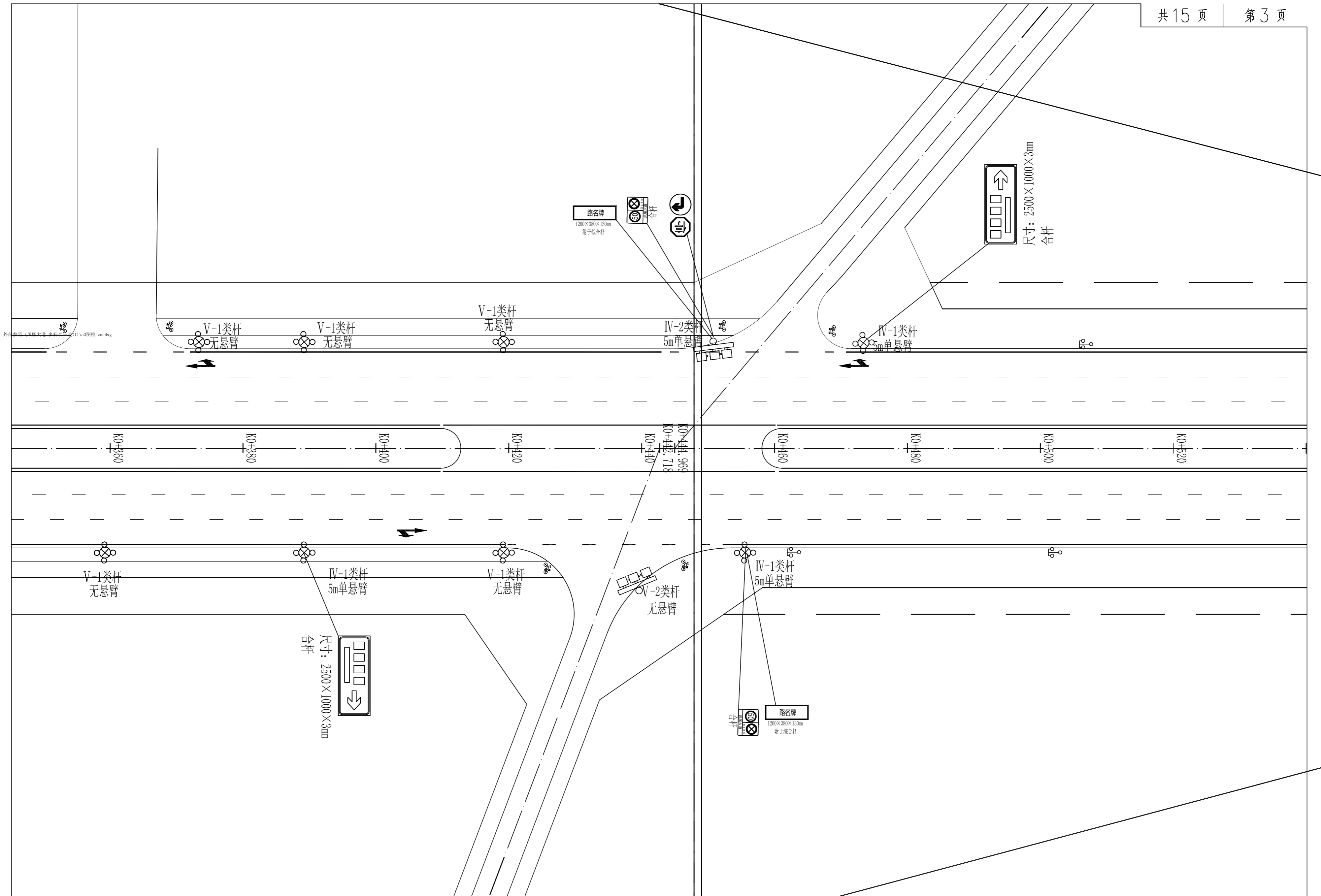
多杆合一平面设计图
